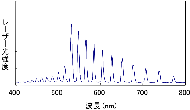
虹色レーザーのスペクトル
